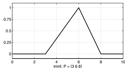
trimf
