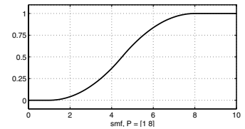
smf
